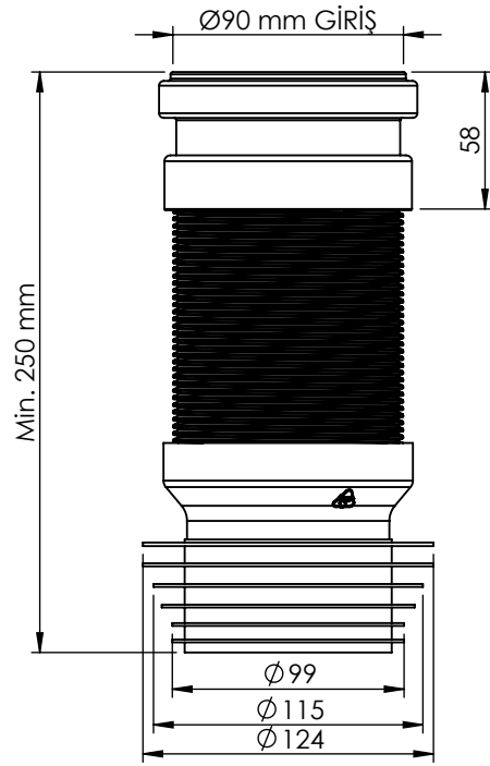
KAPALI POZİSYON
