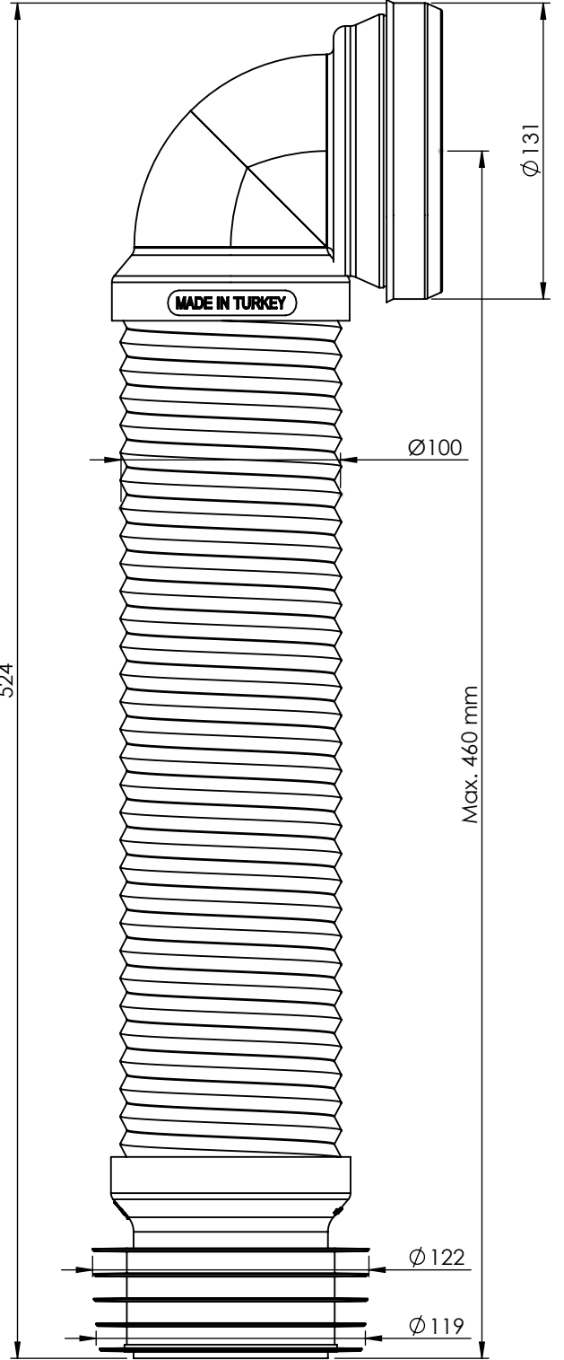
100-110 mm ÇIKIŞ AÇIK POZİSYON
